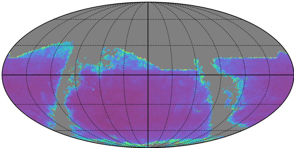
no_long_v3.4_10yrs r band: AGN SF_uncert
