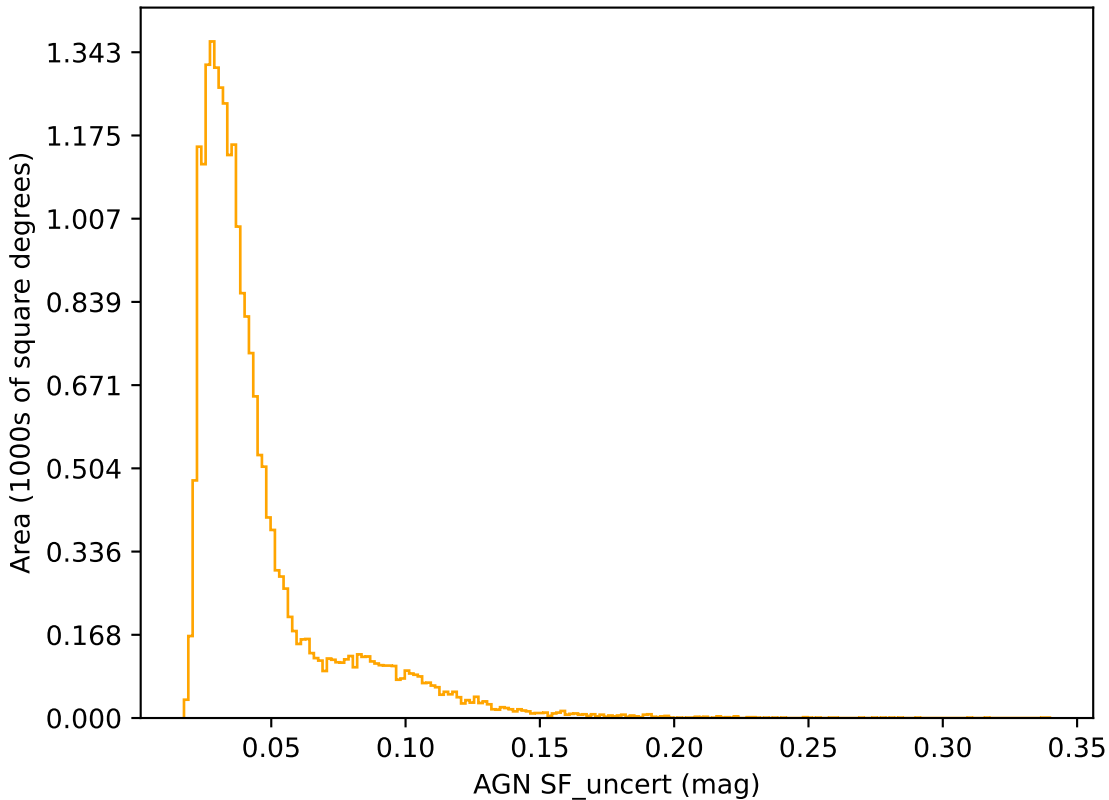
no_long_v3.4_10yrs r band: AGN SF_uncert
