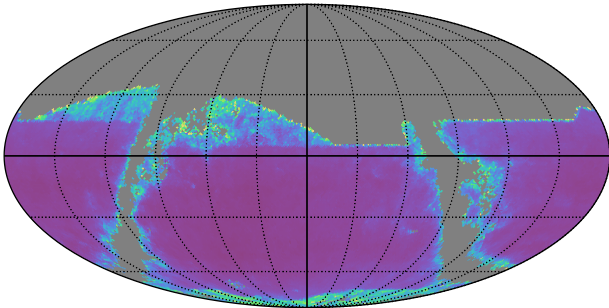
no_long_v3.4_10yrs i band: AGN SF_uncert
