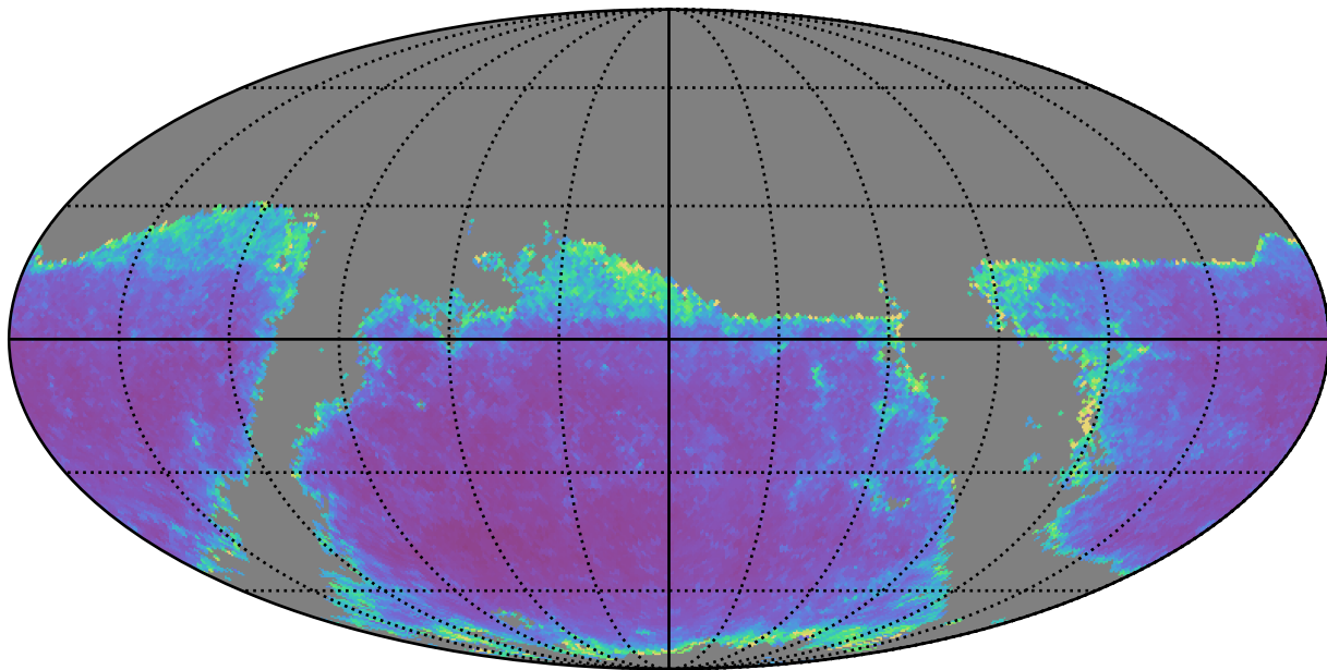
no_long_v3.4_10yrs g band: AGN SF_uncert
