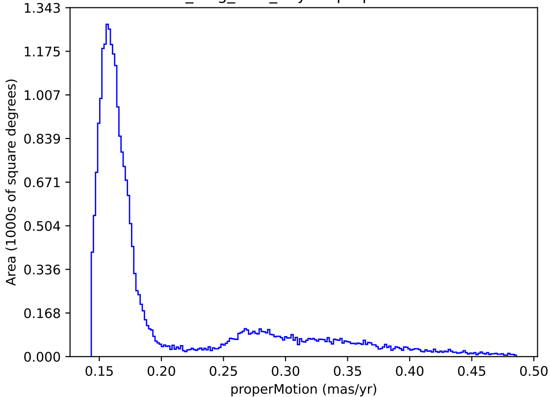
no_long_v3.4_10yrs : properMotion
