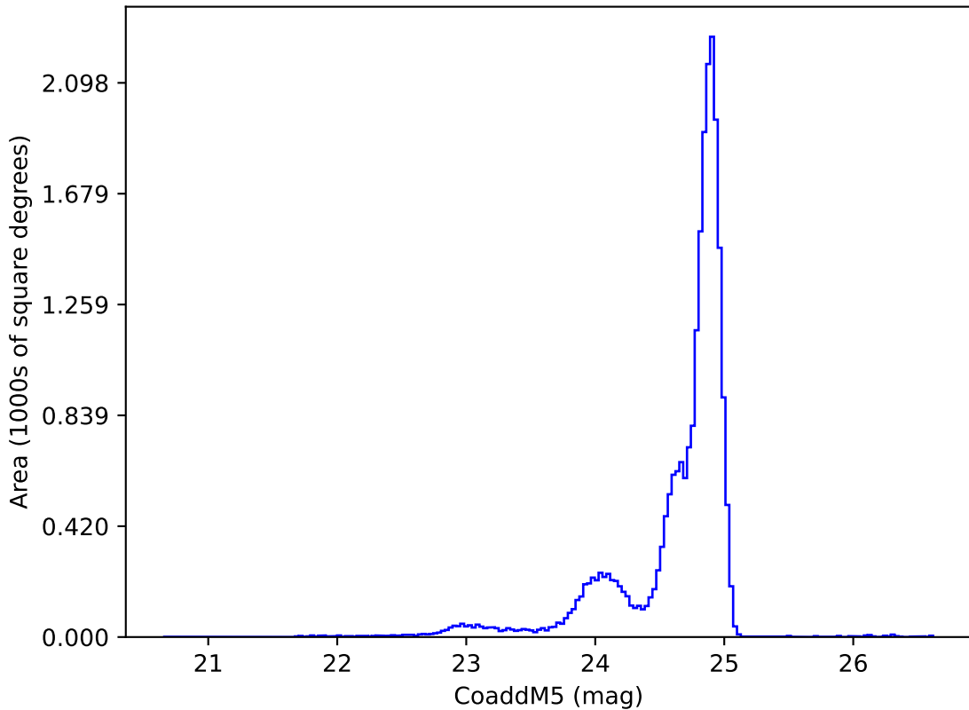
no_long_v3.4_10yrs y: CoaddM5
