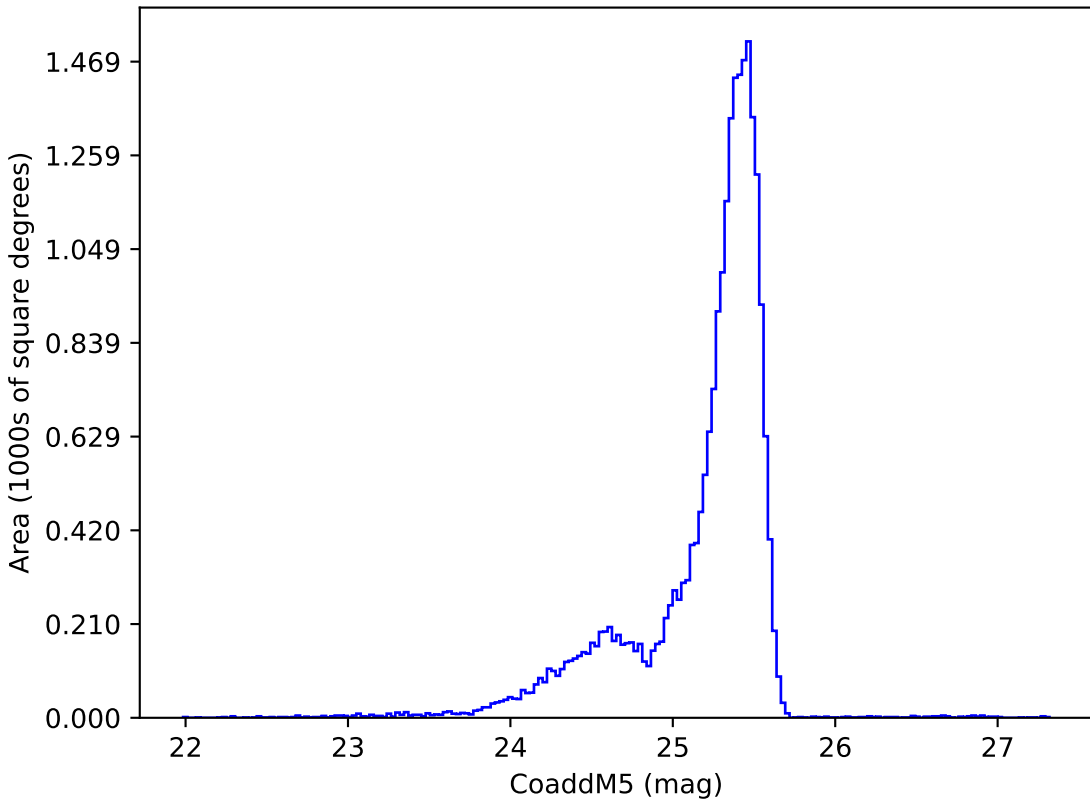
no_long_v3.4_10yrs u: CoaddM5
