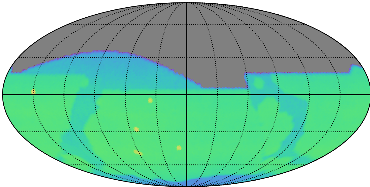
no_long_v3.4_10yrs r: CoaddM5
