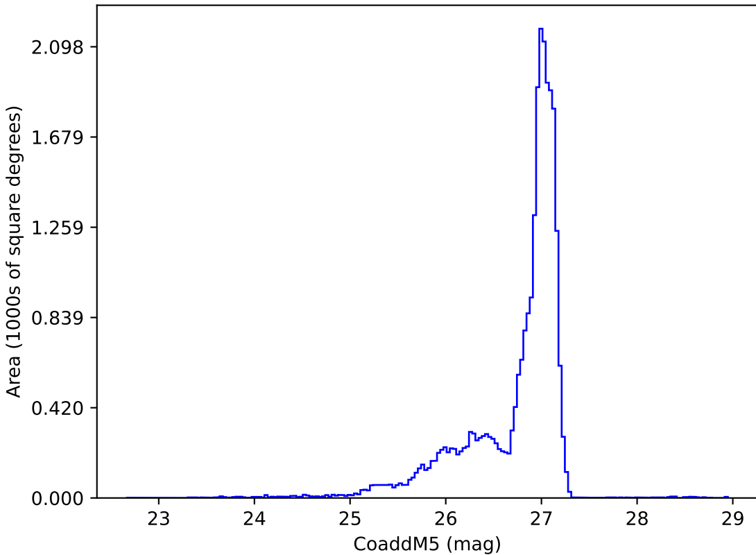
no_long_v3.4_10yrs r: CoaddM5
