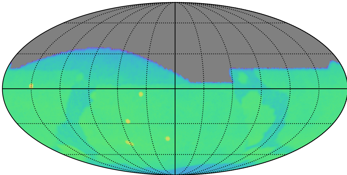
no_long_v3.4_10yrs g: CoaddM5
