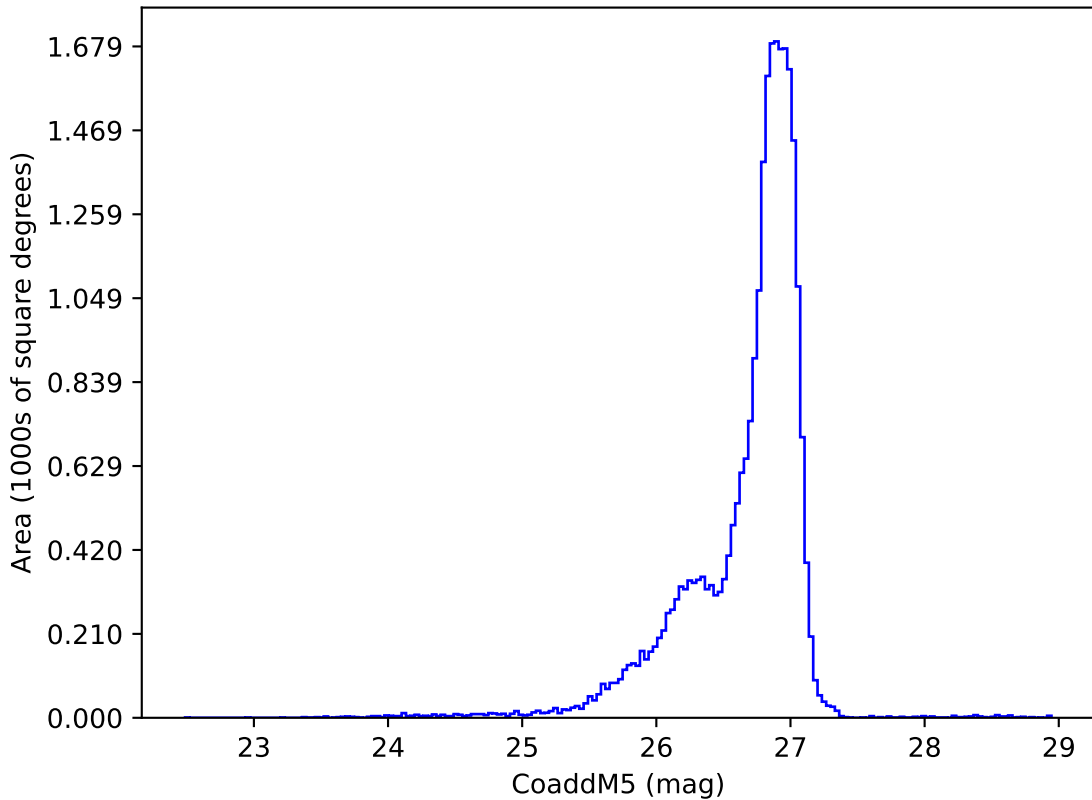
no_long_v3.4_10yrs g: CoaddM5
