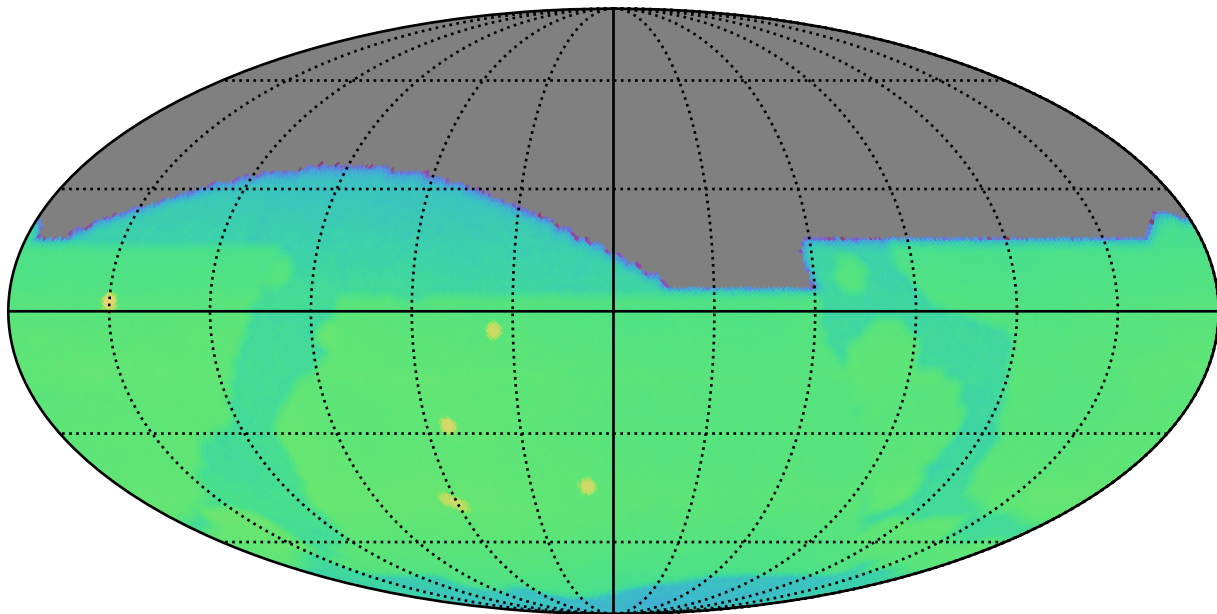
no_long_v3.4_10yrs : CoaddM5
