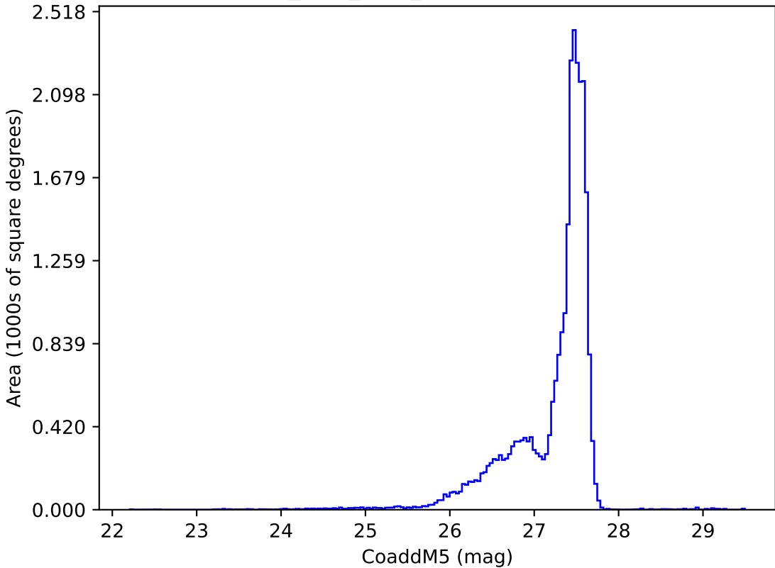
no_long_v3.4_10yrs : CoaddM5
