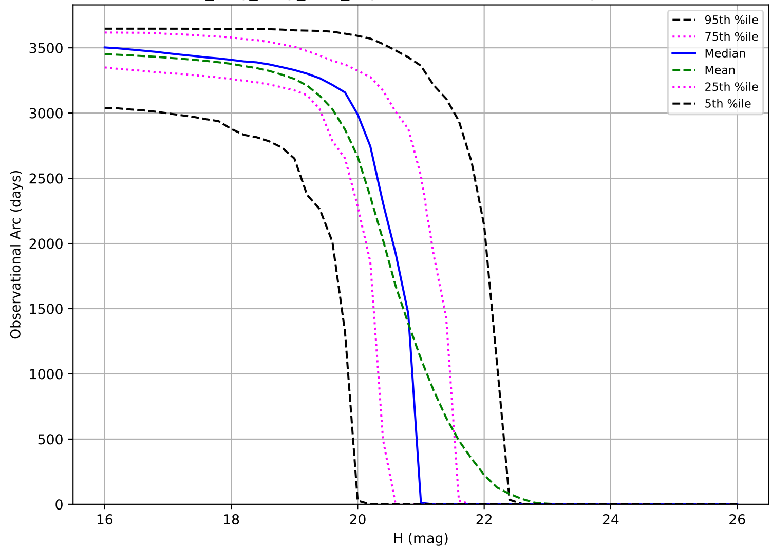
no_long_daily_v3.4_10yrs: Observational Arc Length MBA
