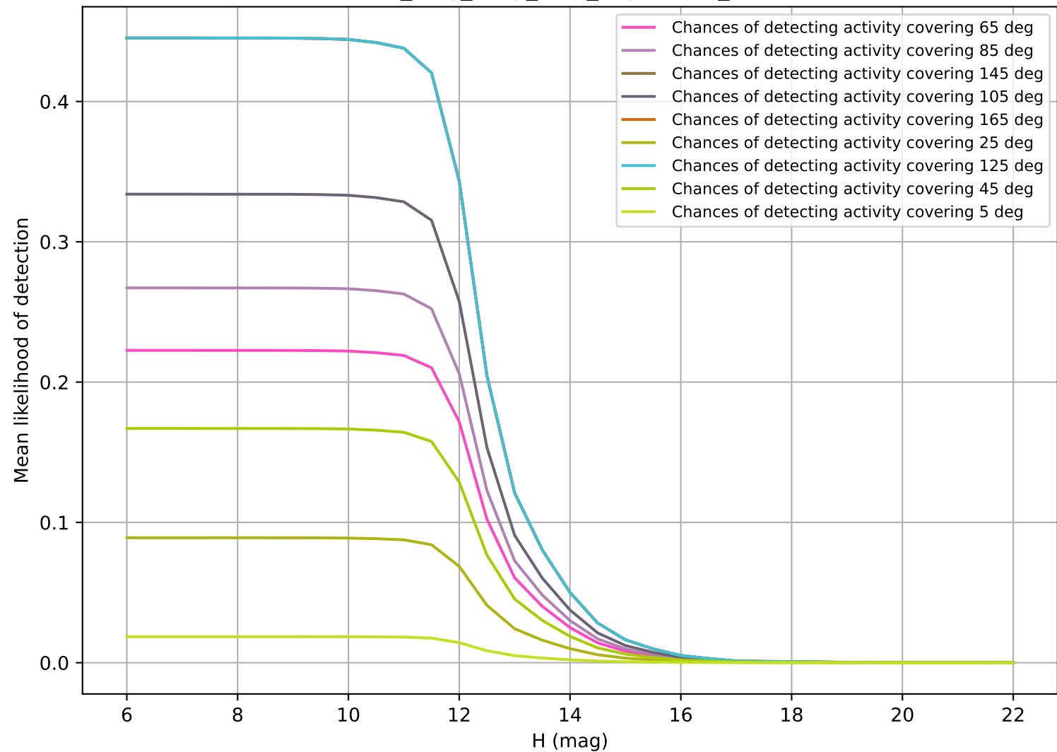
no_long_daily_v3.4_10yrs OCC_r20
