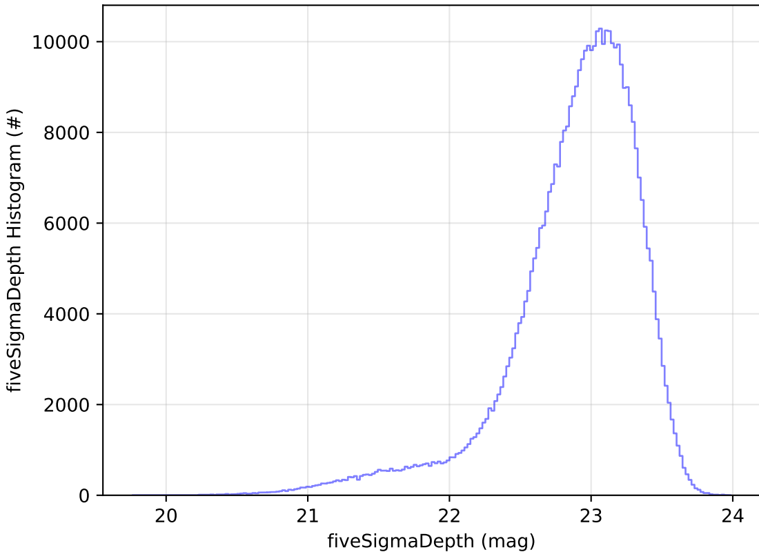
no_long_daily_v3.4_10yrs z: fiveSigmaDepth Histogram
