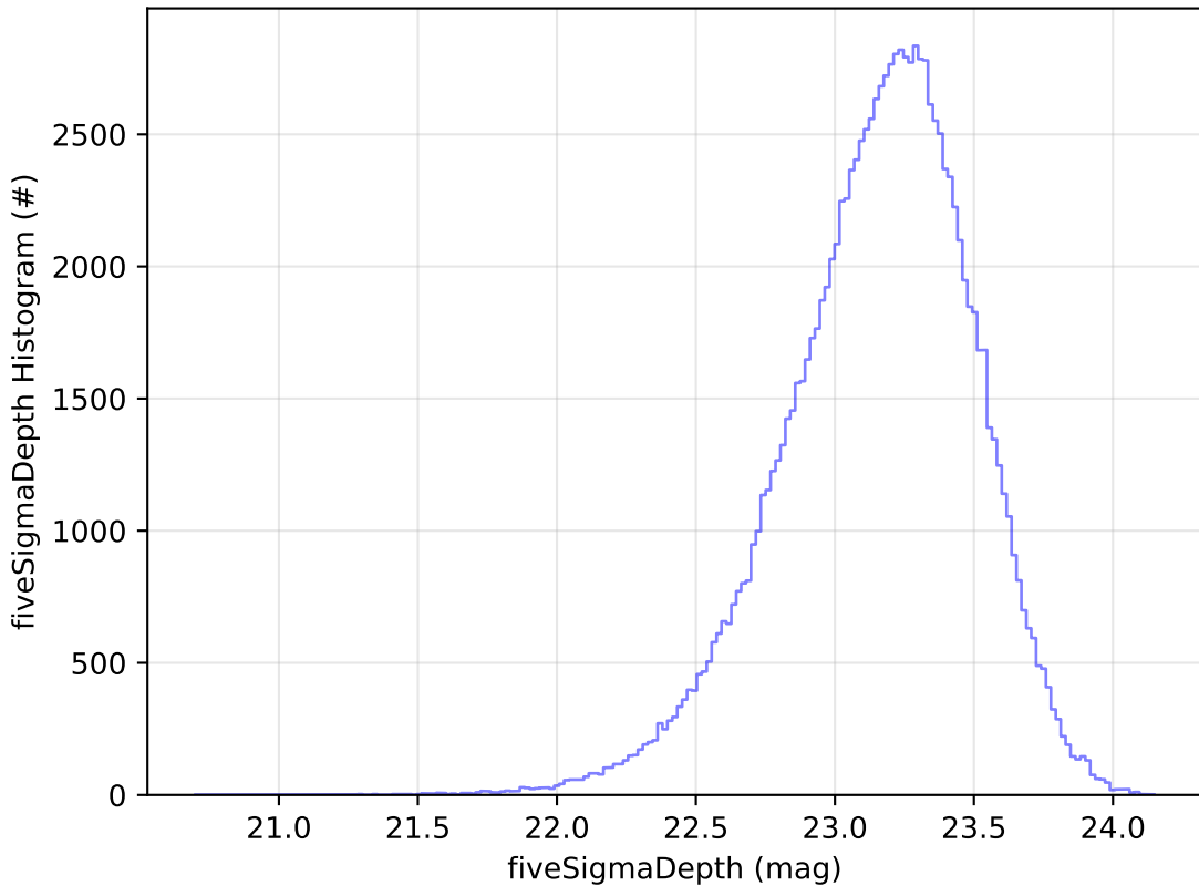
no_long_daily_v3.4_10yrs u: fiveSigmaDepth Histogram
