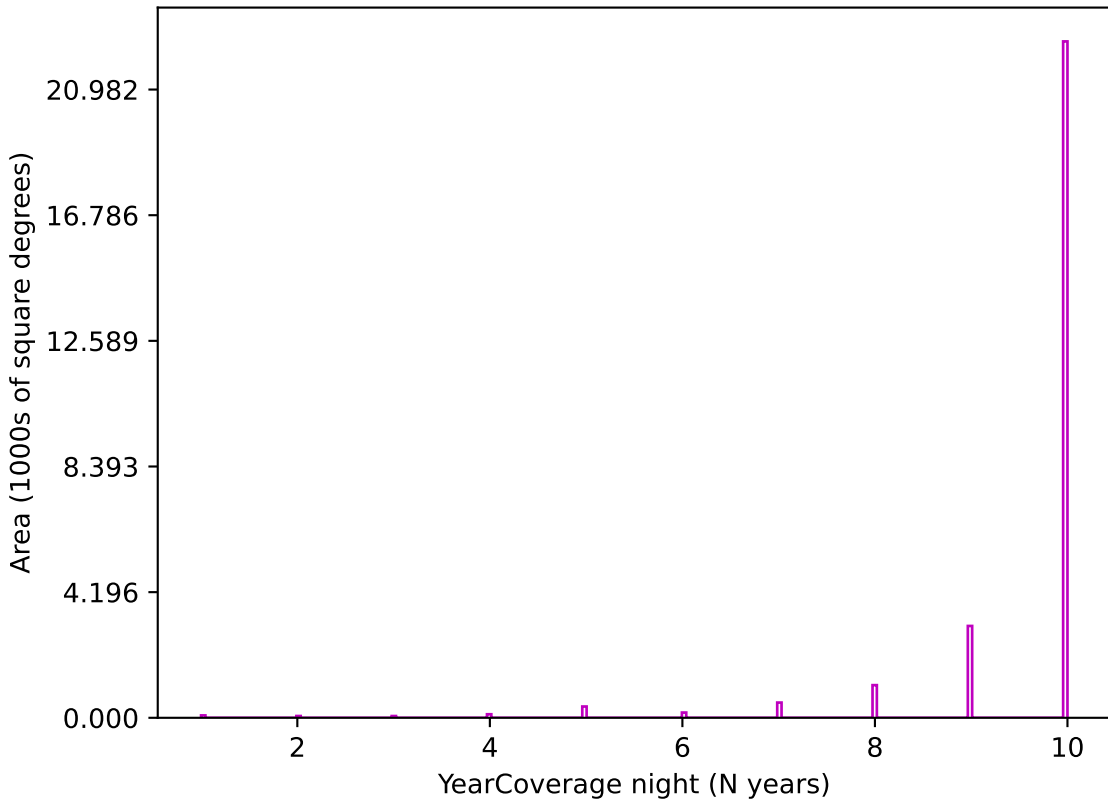
no_long_daily_v3.4_10yrs z band: YearCoverage night
