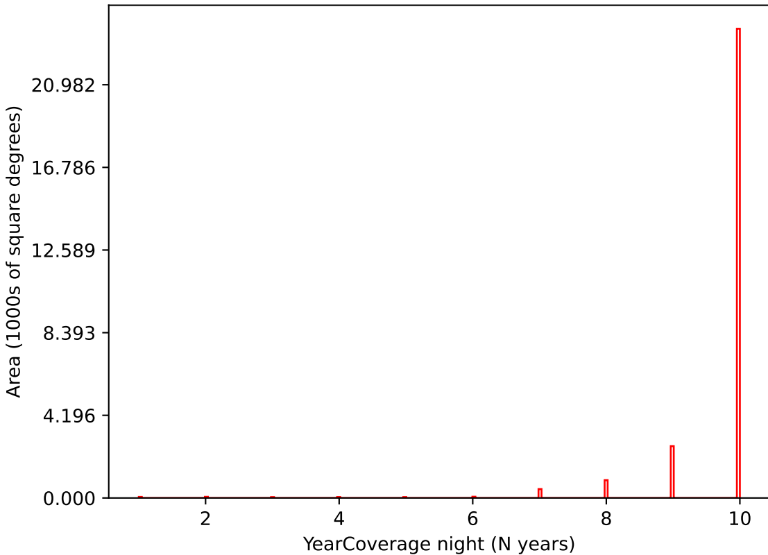
no_long_daily_v3.4_10yrs i band: YearCoverage night
