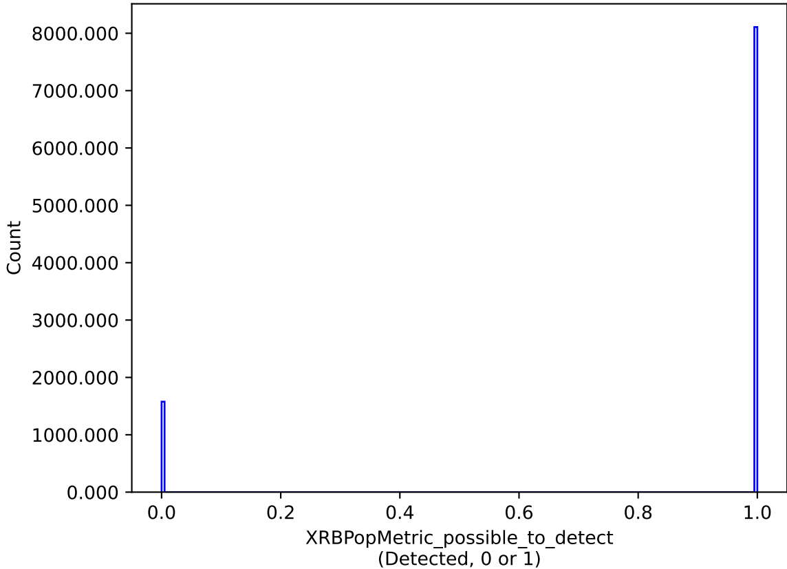
no_long_daily_v3.4_10yrs : XRBPoMetric_possible_to_detect
