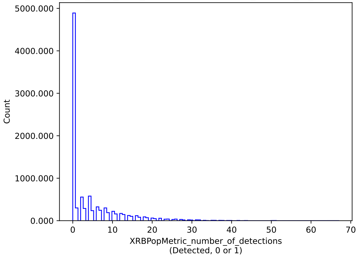
no_long_daily_v3.4_10yrs : XRBPoMetric_number_of_detections
