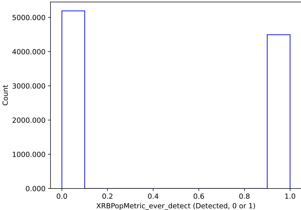
no_long_daily_v3.4_10yrs : XRBPoMetric_ever_detect
