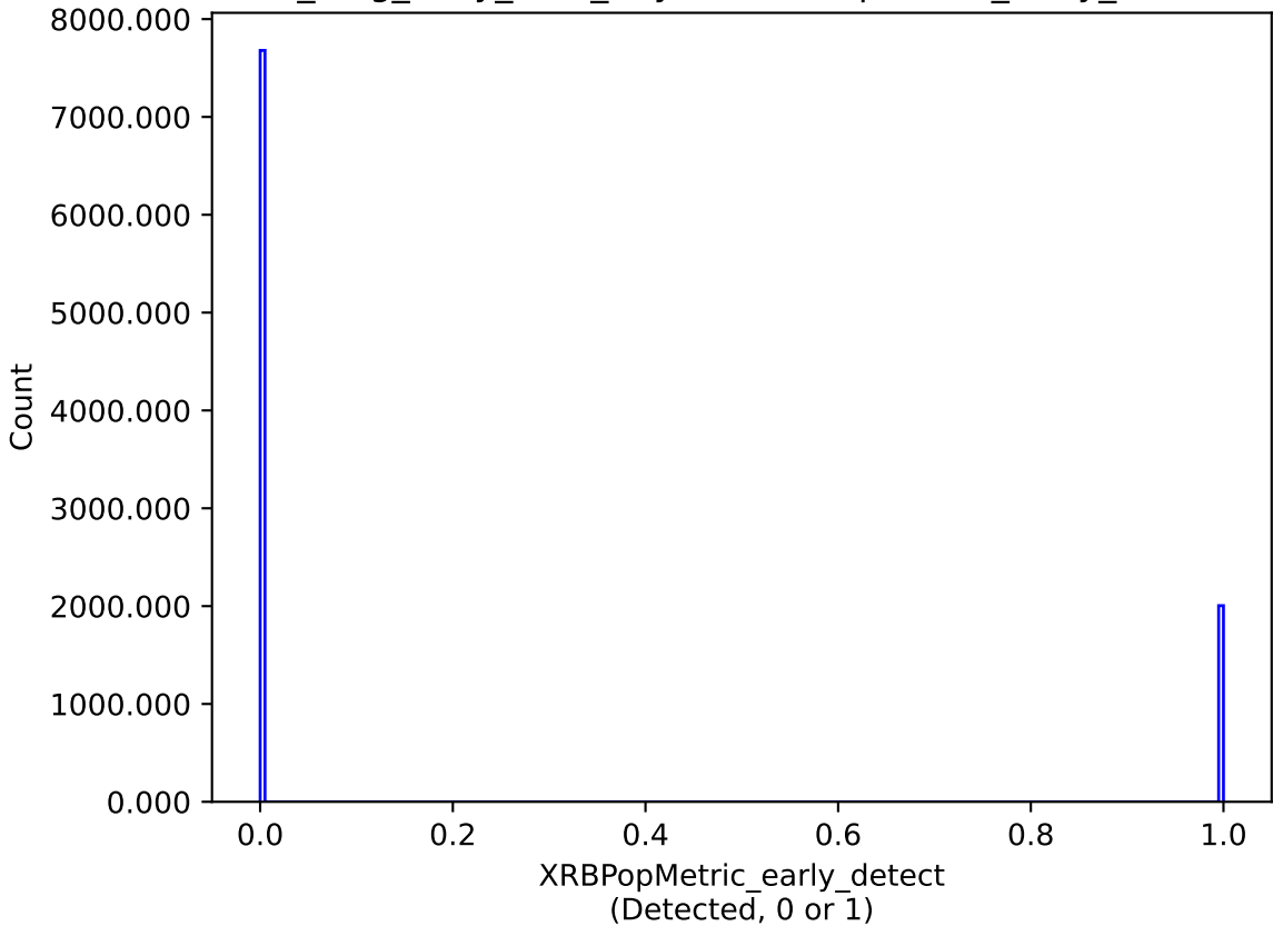
no_long_daily_v3.4_10yrs : XRBPoMetric_early_detect
