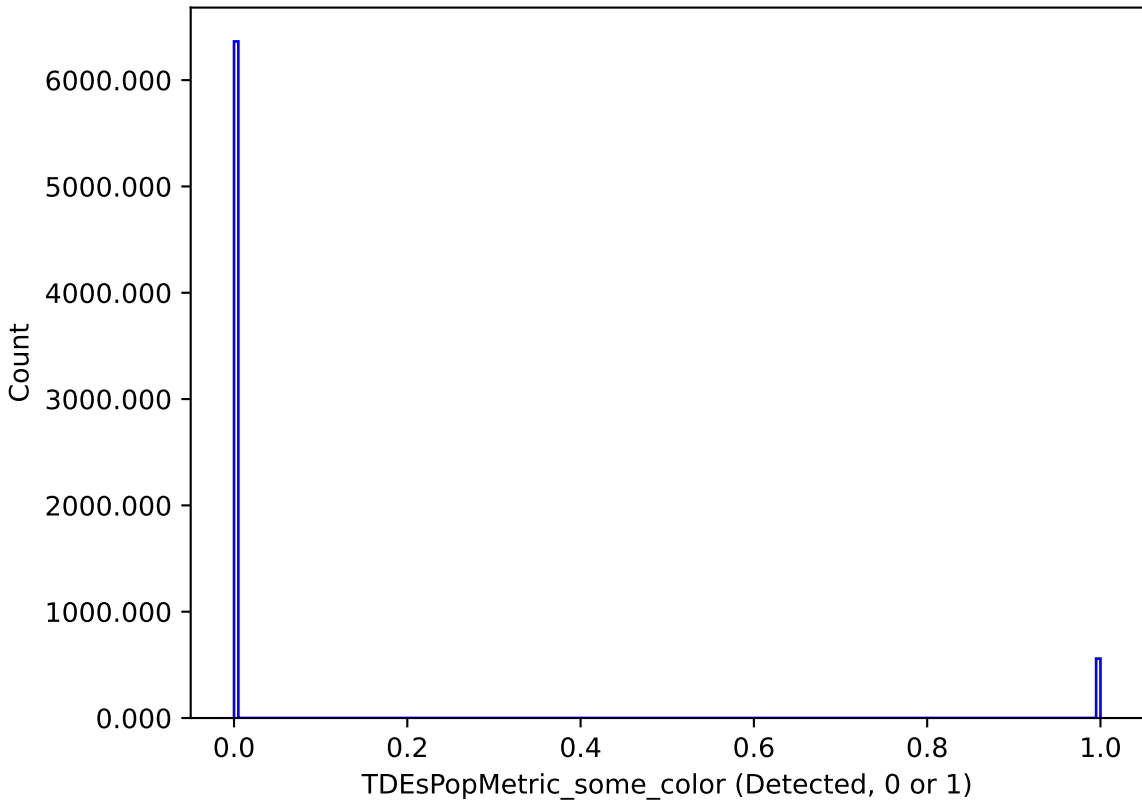
no_long_daily_v3.4_10yrs : TDEsPopMetric_some_color
