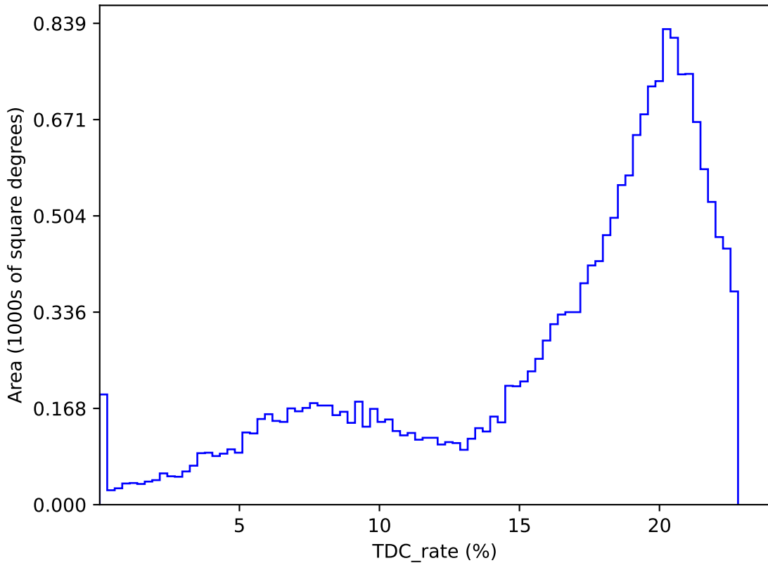
no_long_daily_v3.4_10yrs : TDC_rate
