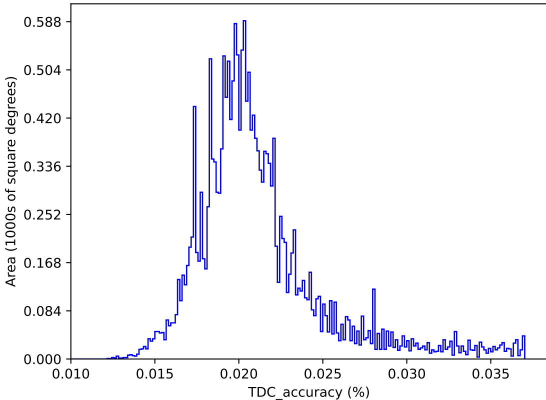
no_long_daily_v3.4_10yrs : TDC_accuracy
