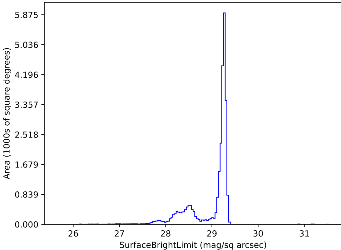
no_long_daily_v3.4_10yrs z: SurfaceBrightLimit
