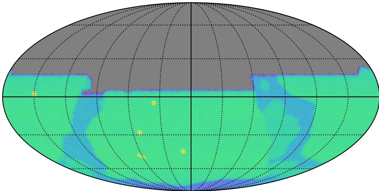
no_long_daily_v3.4_10yrs y: SurfaceBrightLimit
