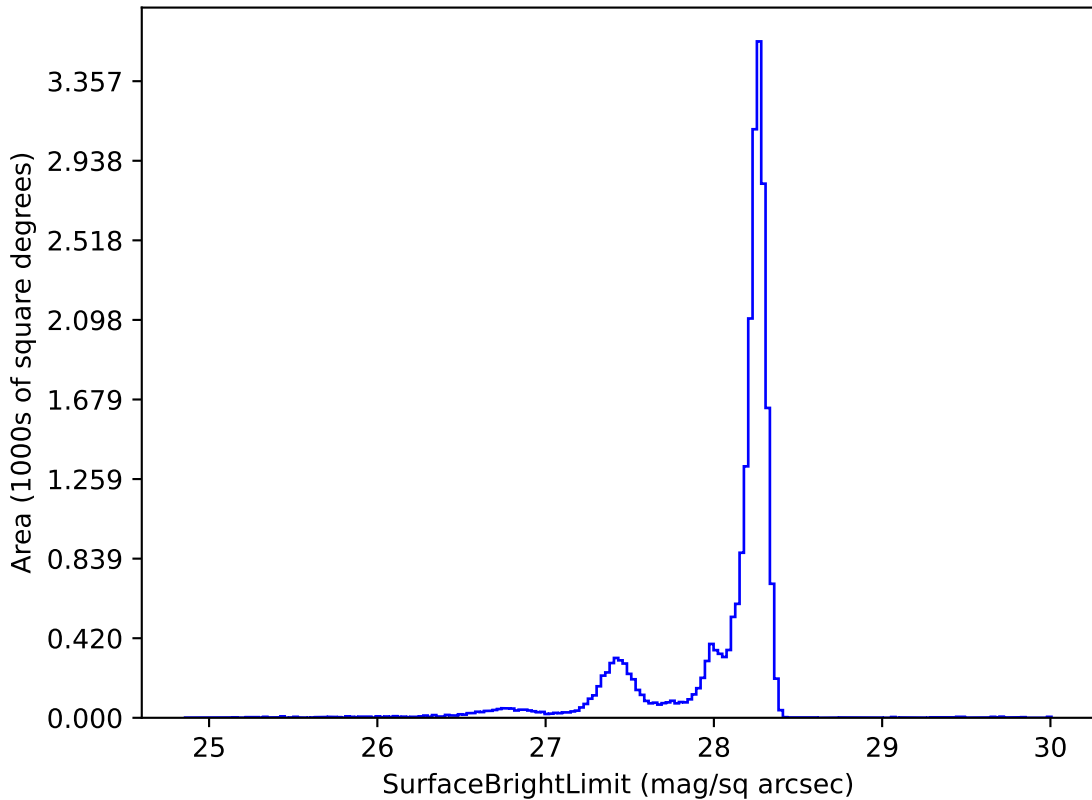
no_long_daily_v3.4_10yrs y: SurfaceBrightLimit
