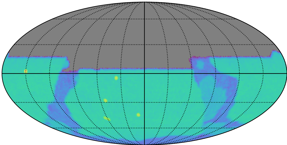
no_long_daily_v3.4_10yrs u: SurfaceBrightLimit
