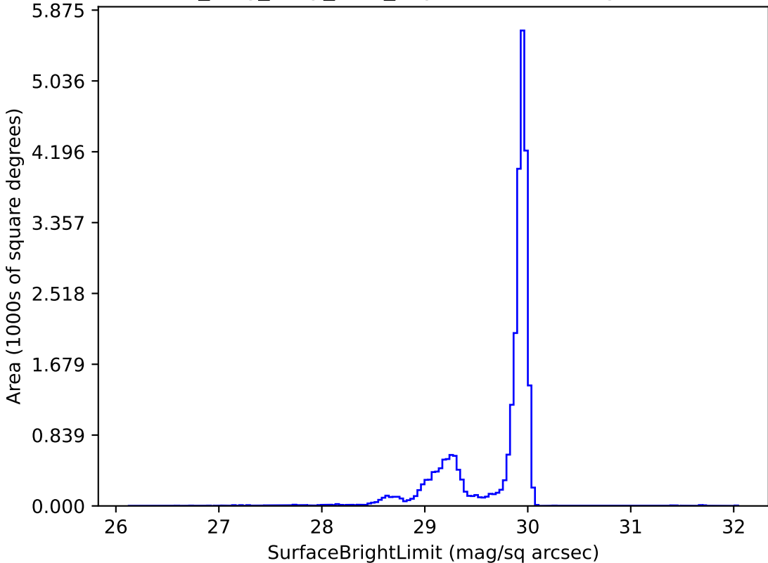
no_long_daily_v3.4_10yrs i: SurfaceBrightLimit
