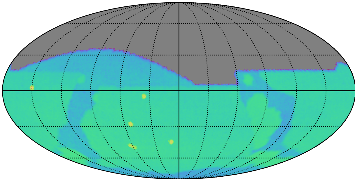
no_long_daily_v3.4_10yrs g: SurfaceBrightLimit
