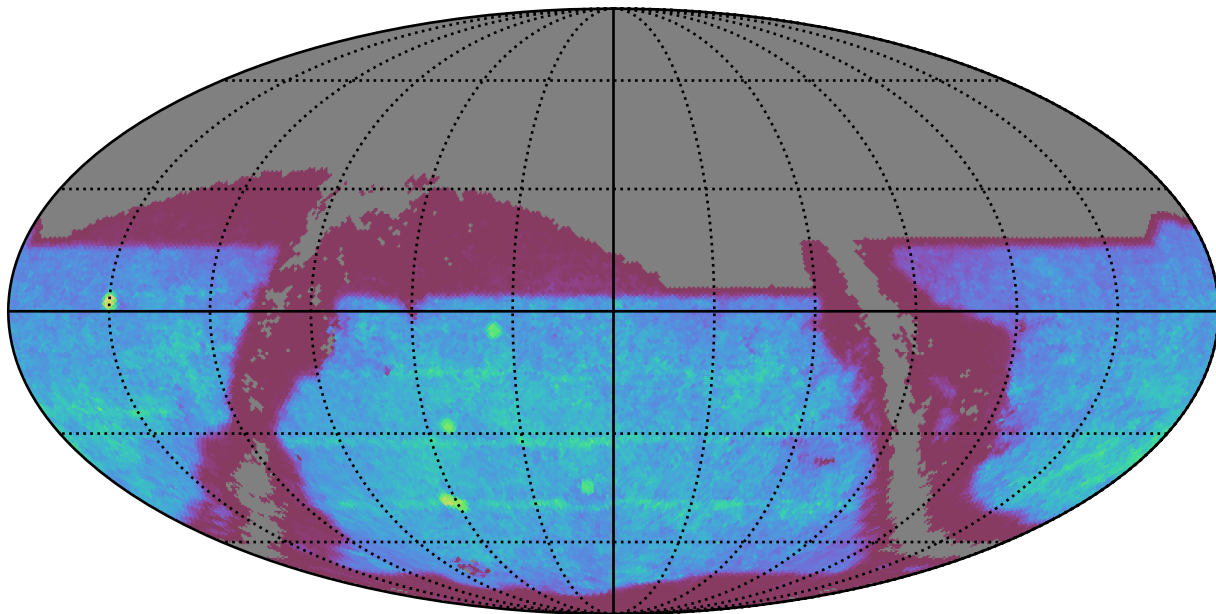
no_long_daily_v3.4_10yrs : SNSLMetric
