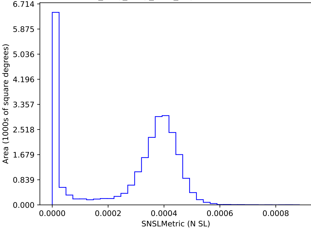
no_long_daily_v3.4_10yrs : SNSLMetric
