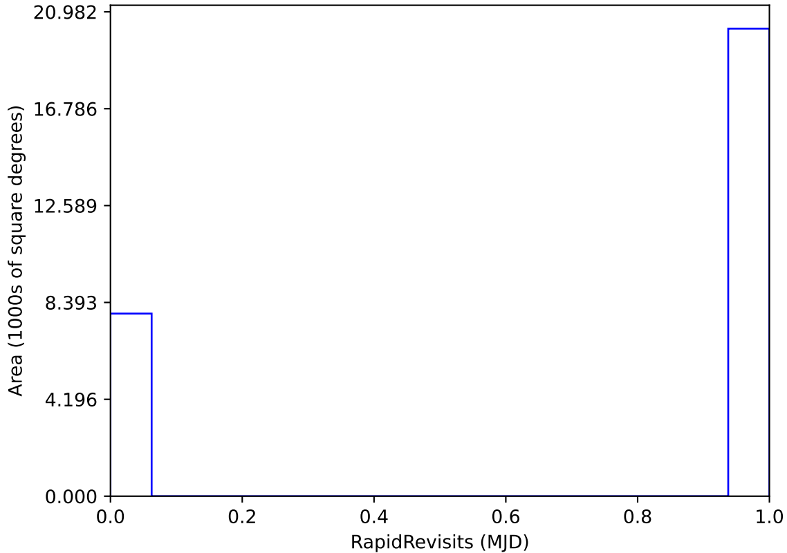
no_long_daily_v3.4_10yrs : RapidRevisits
