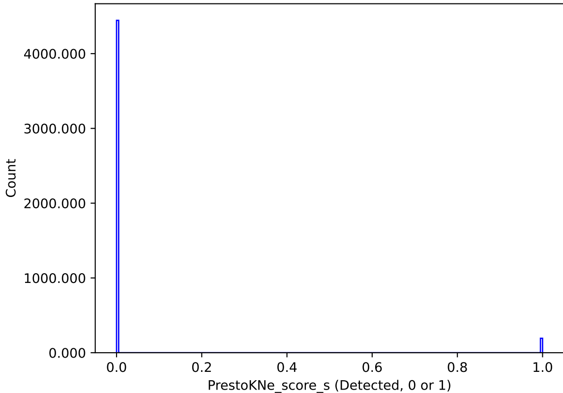
no_long_daily_v3.4_10yrs : PrestoKNe_score_s
