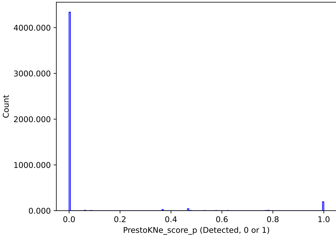
no_long_daily_v3.4_10yrs : PrestoKNe_score_p
