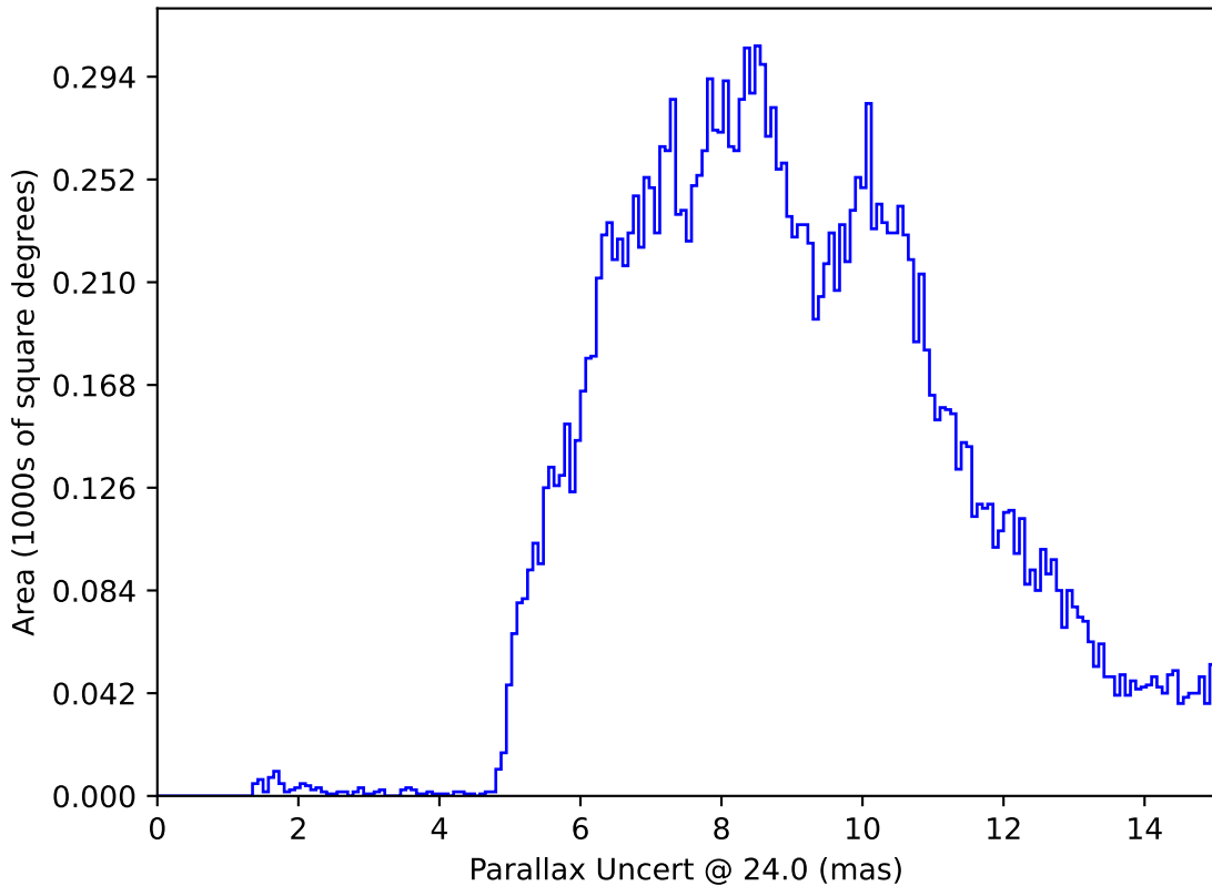
no_long_daily_v3.4_10yrs : Parallax Uncert @ 24.0
