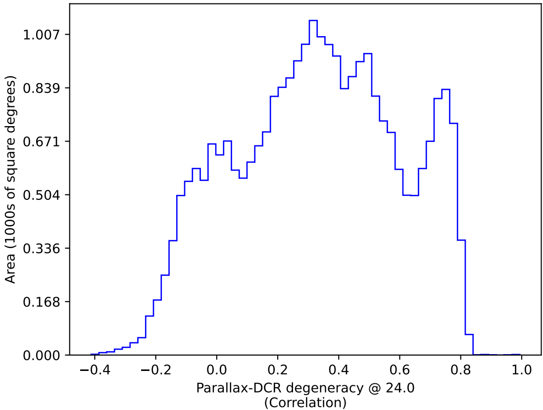
no_long_daily_v3.4_10yrs : Parallax-DCR degeneracy @ 24.0
