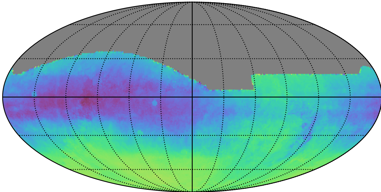
no_long_daily_v3.4_10yrs : Parallax-DCR degeneracy @ 22.4
