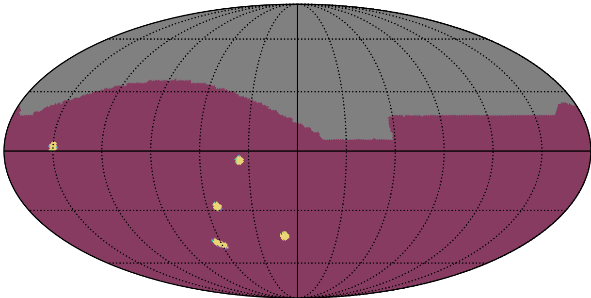
no_long_daily_v3.4_10yrs : NumberOfQuickRevisits
