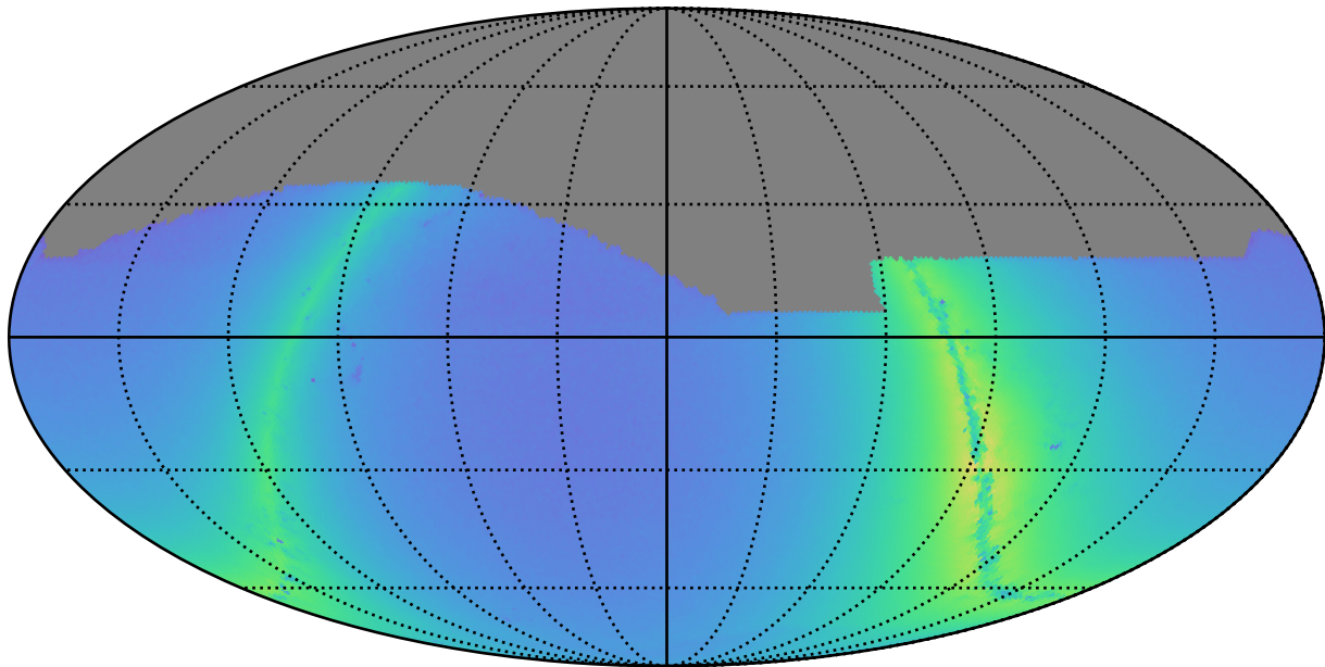
no_long_daily_v3.4_10yrs z: Nstars_no_crowding
