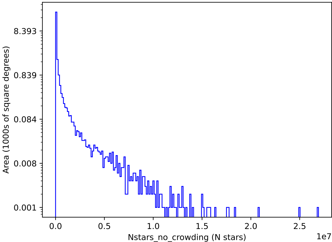
no_long_daily_v3.4_10yrs z: Nstars_no_crowding
