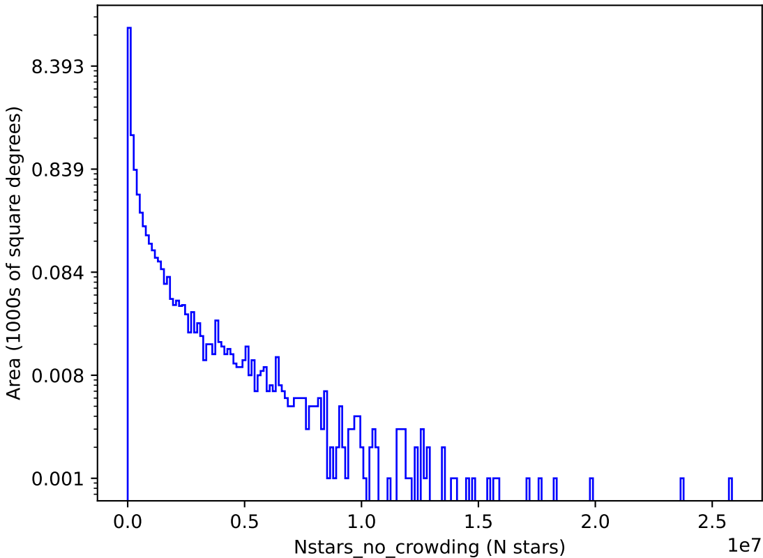
no_long_daily_v3.4_10yrs y: Nstars_no_crowding
