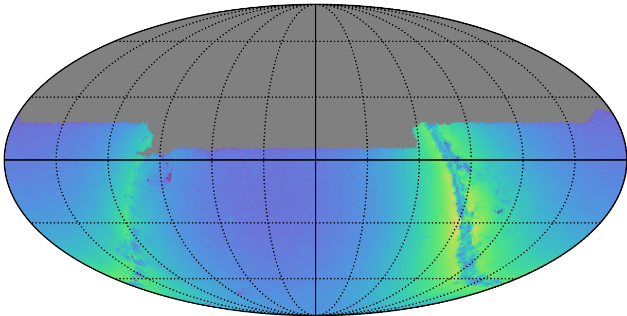
no_long_daily_v3.4_10yrs u: Nstars_no_crowding
