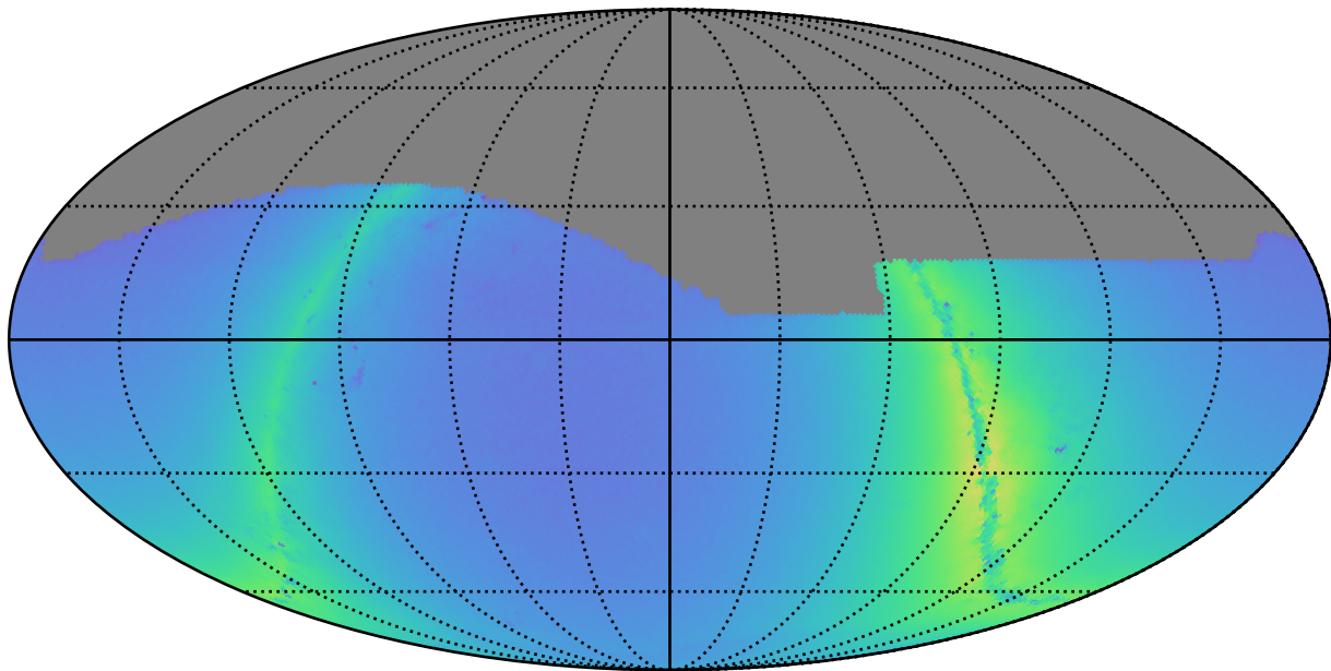
no_long_daily_v3.4_10yrs r: Nstars_no_crowding
