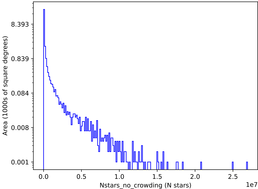
no_long_daily_v3.4_10yrs i: Nstars_no_crowding
