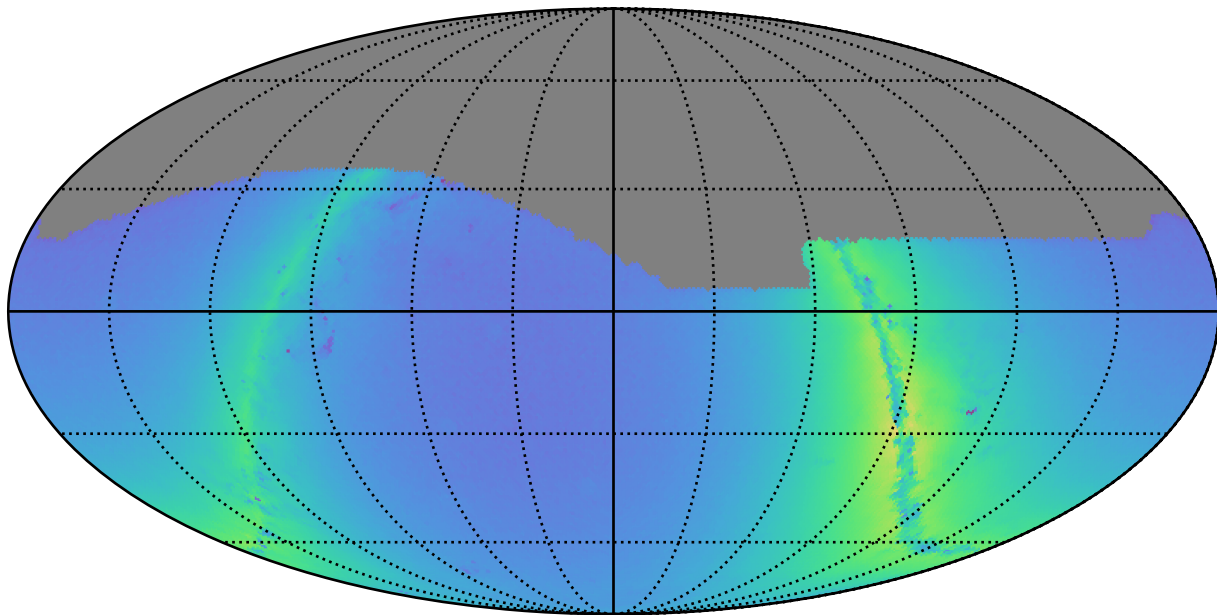
no_long_daily_v3.4_10yrs g: Nstars_no_crowding
