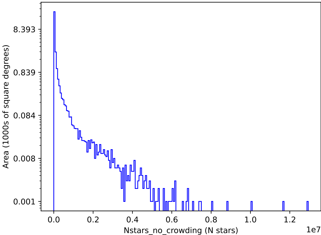
no_long_daily_v3.4_10yrs g: Nstars_no_crowding
