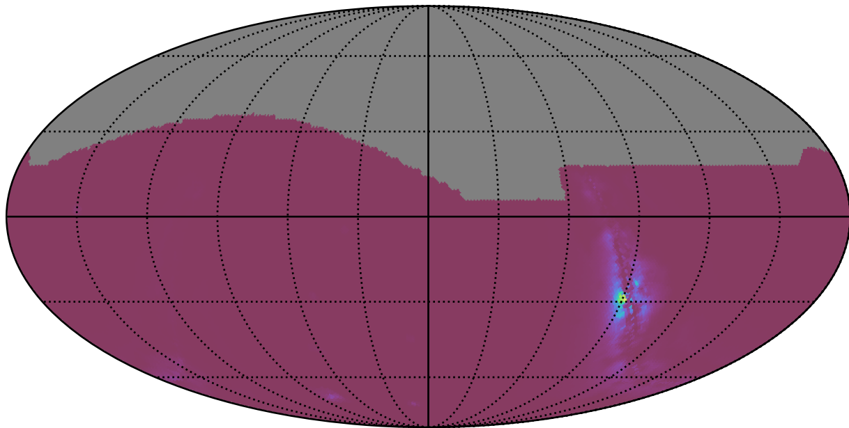
no_long_daily_v3.4_10yrs : NlcPoints
